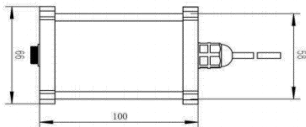
分体板尺寸图
